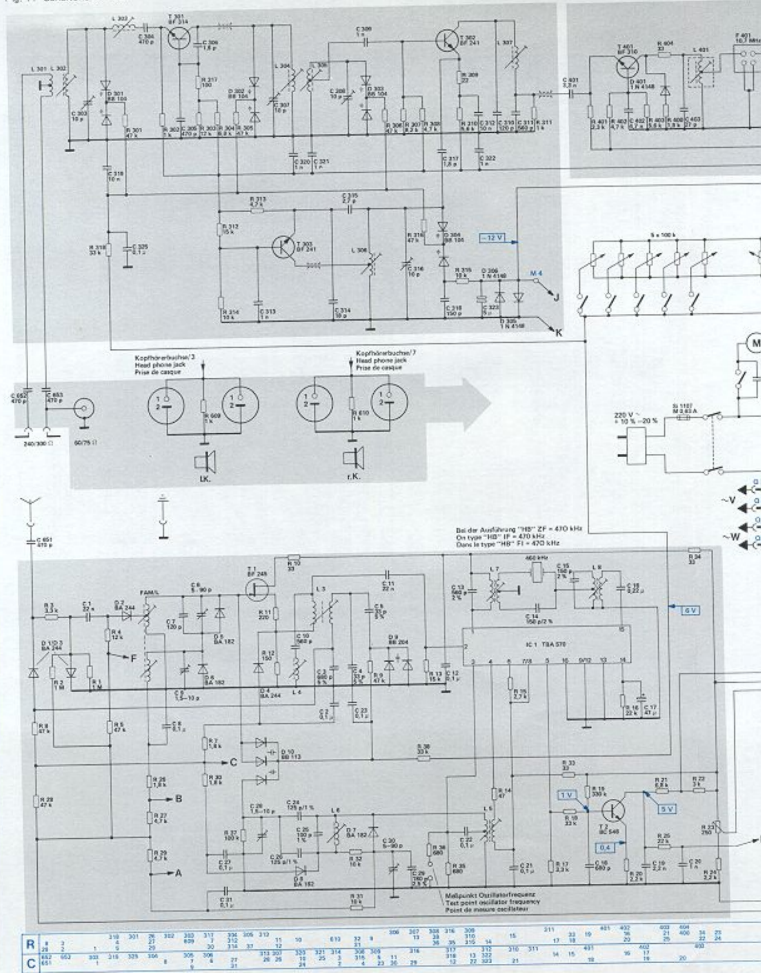
Fig. 11 Schaltbild HF-Teil
